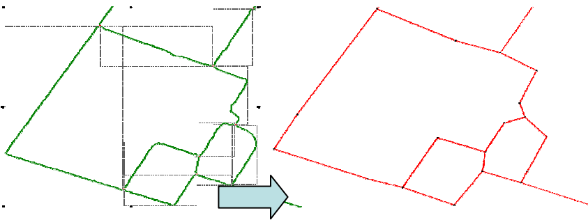
Vectorisation
